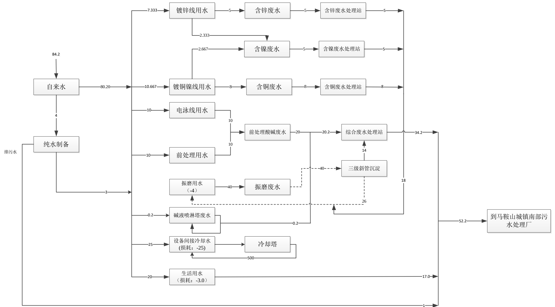
图 2-13 现有项目水平衡图 (单位: \text{m}^3/\text{d} )
