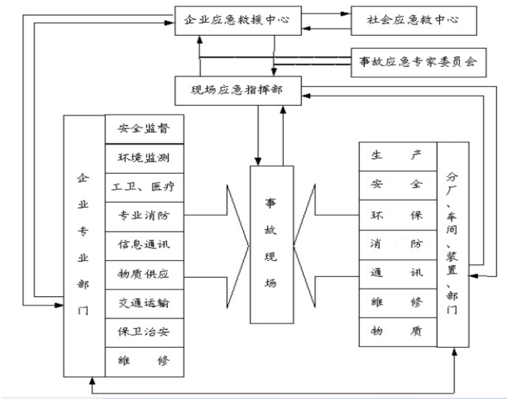
图 6-3 企业风险事故应急组织系统基本框图
