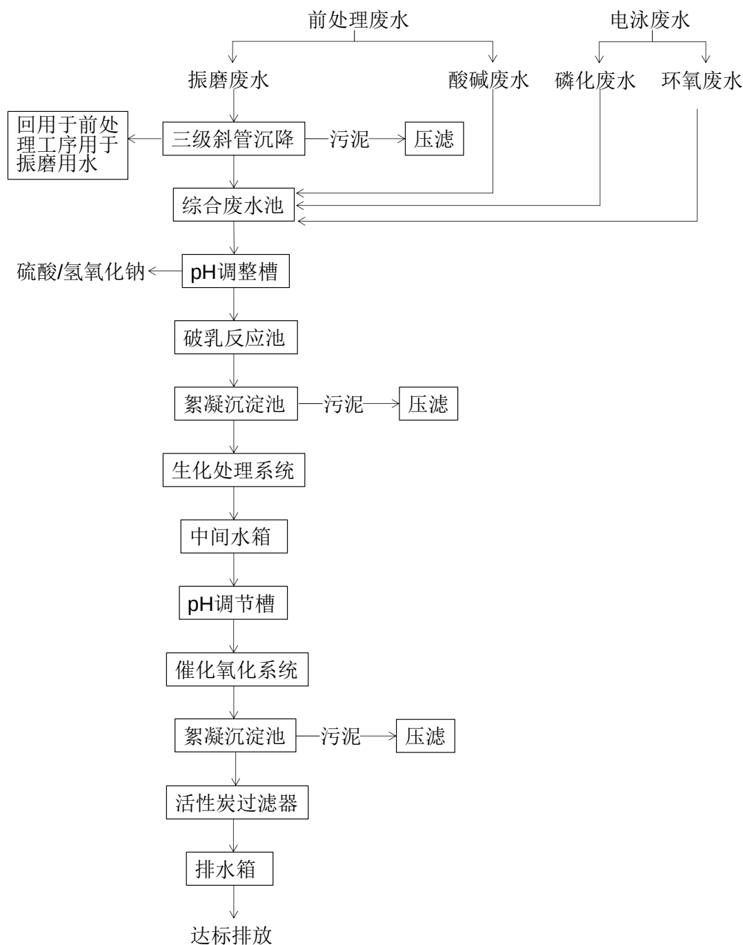
图 7-5 综合废水处理工艺
