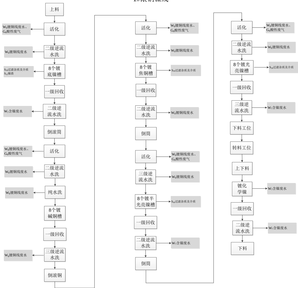
图 3-19 1#滚铜镍线工艺流程及产污环节图
