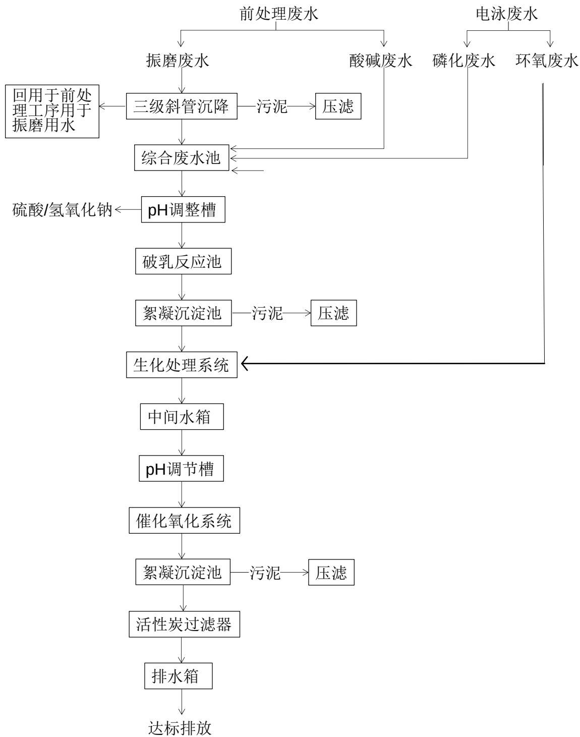
图 2-11 综合废水处理工艺
