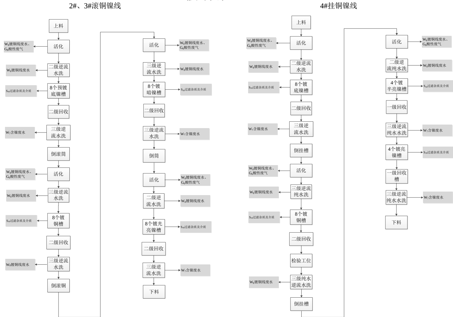
图 3-20 2#、3#滚铜镍线，4#挂铜镍线工艺流程及产污环节图
