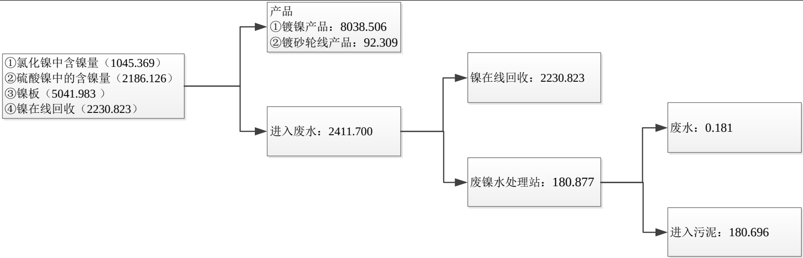
图 3-11 镍元素平衡图（单位：kg/a）
