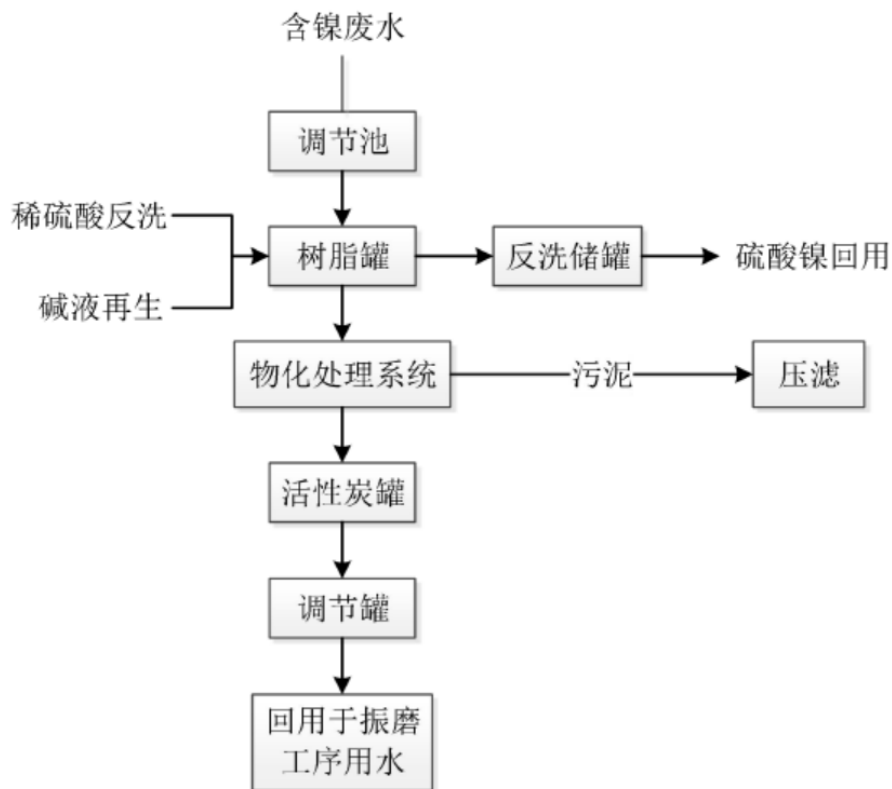
图 2-10 含镍废水处理工艺
