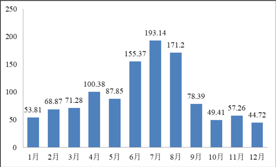
图 5-3 马鞍山累年月平均降水量（单位：毫米）
