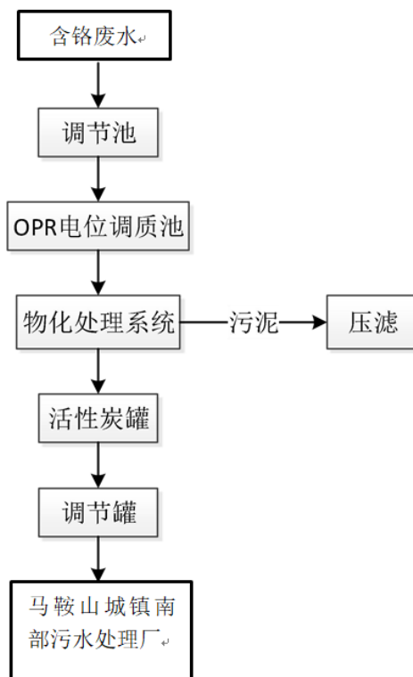
图 7-4 含铬废水处理工艺流程
