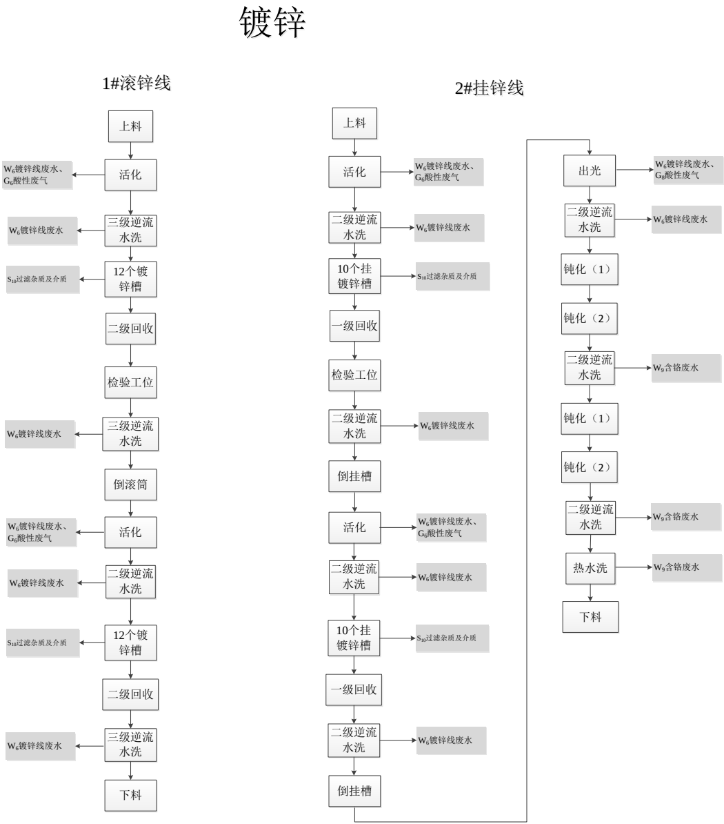
图 3-17 镀锌线工艺流程及产污环节图
