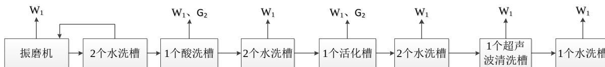
图 2-3 前处理工艺流程及产污环节图
