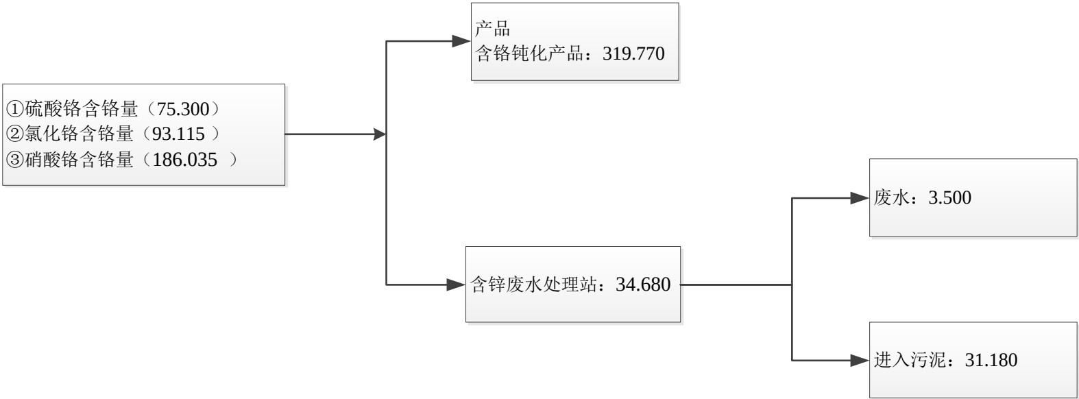
图 3-14 铬元素平衡图（单位：kg/a）
