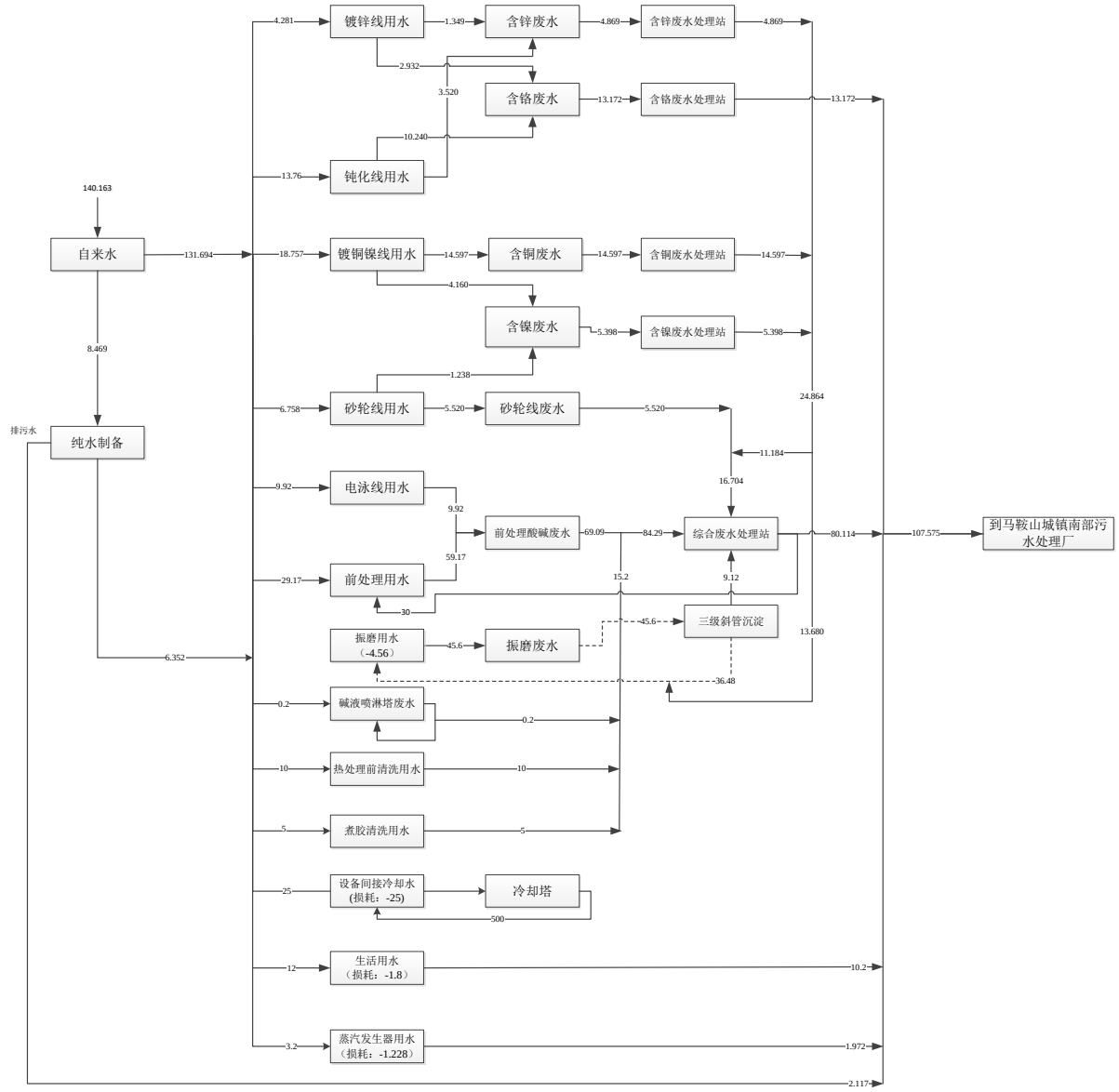
图 3-9 改扩建项目水平衡图 (t/d)
