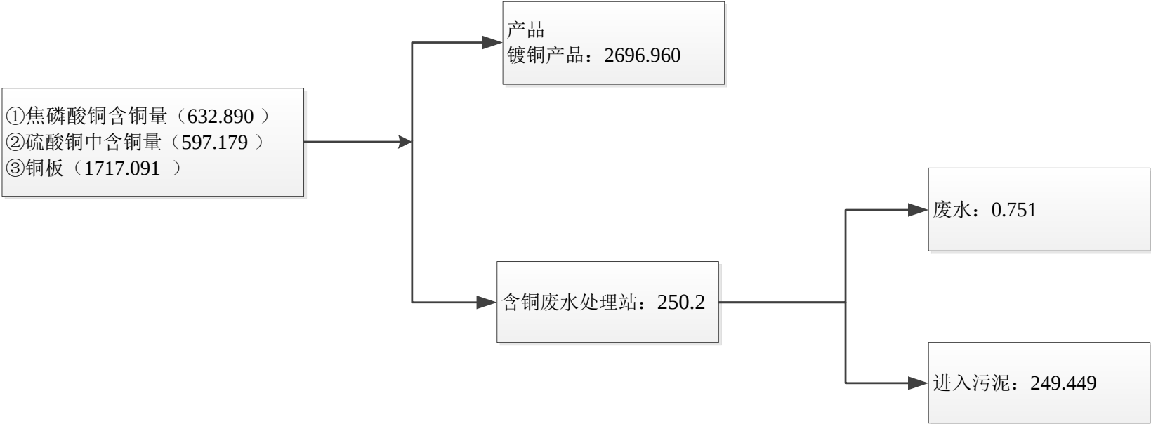
图 3-12 铜元素平衡图（单位：kg/a）
