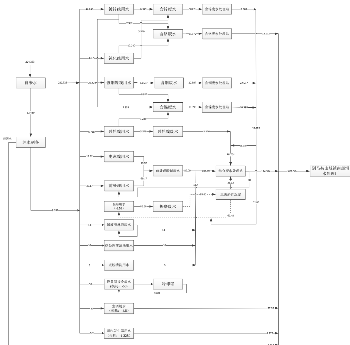
图 3-10 改扩建项目实施后全厂水平衡图 (t/d)
