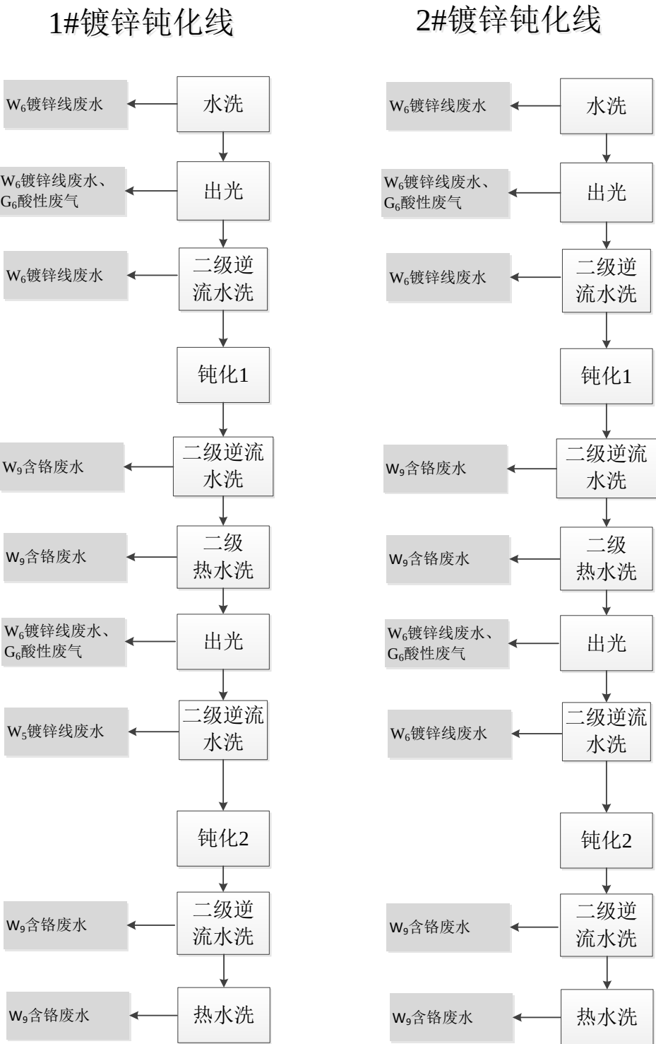
图 3-18 镀锌钝化后处理工艺流程及产污环节
