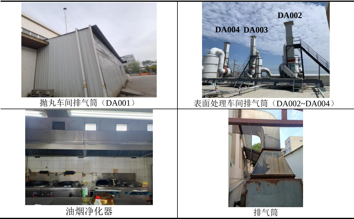
图 2-7 公司厂区现有废气治理设施图片
