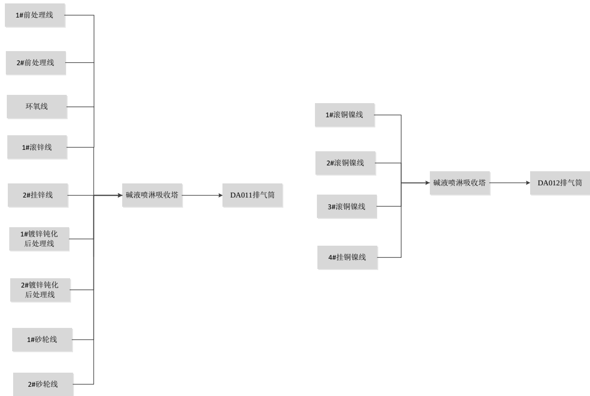
图 7-2 酸雾收集处理方式图
