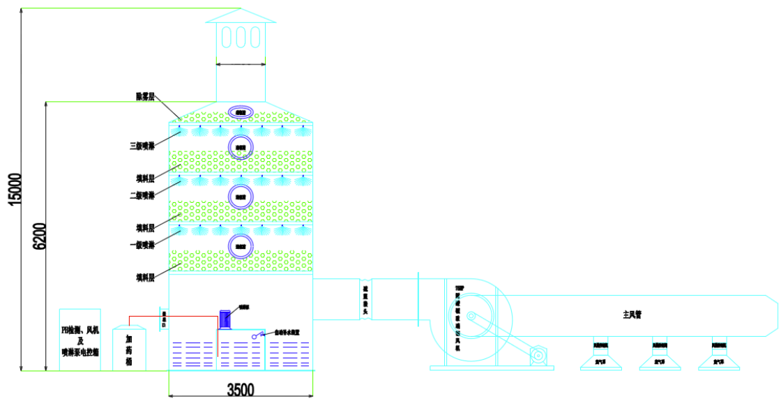
图 7-3 碱液喷淋吸收塔示意图
