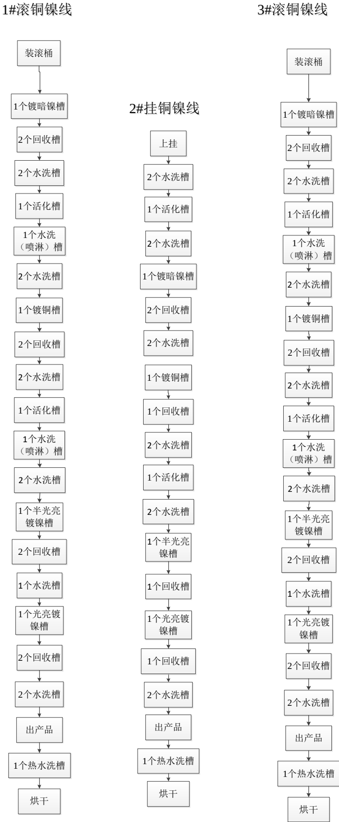
图 2-5 镀铜镍生产线生产工艺
