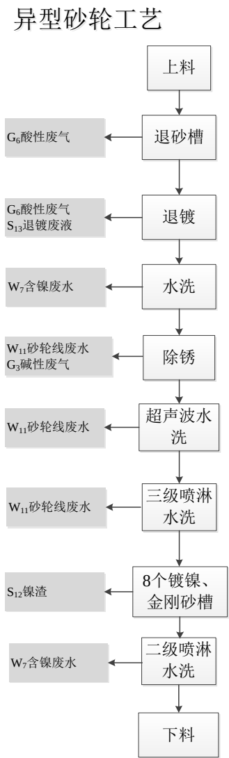
图 3-22 异型砂轮线工艺及产污环节见图
