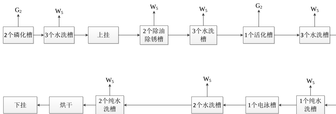
图 2-6 电泳工序生产工艺及产污环节见图
