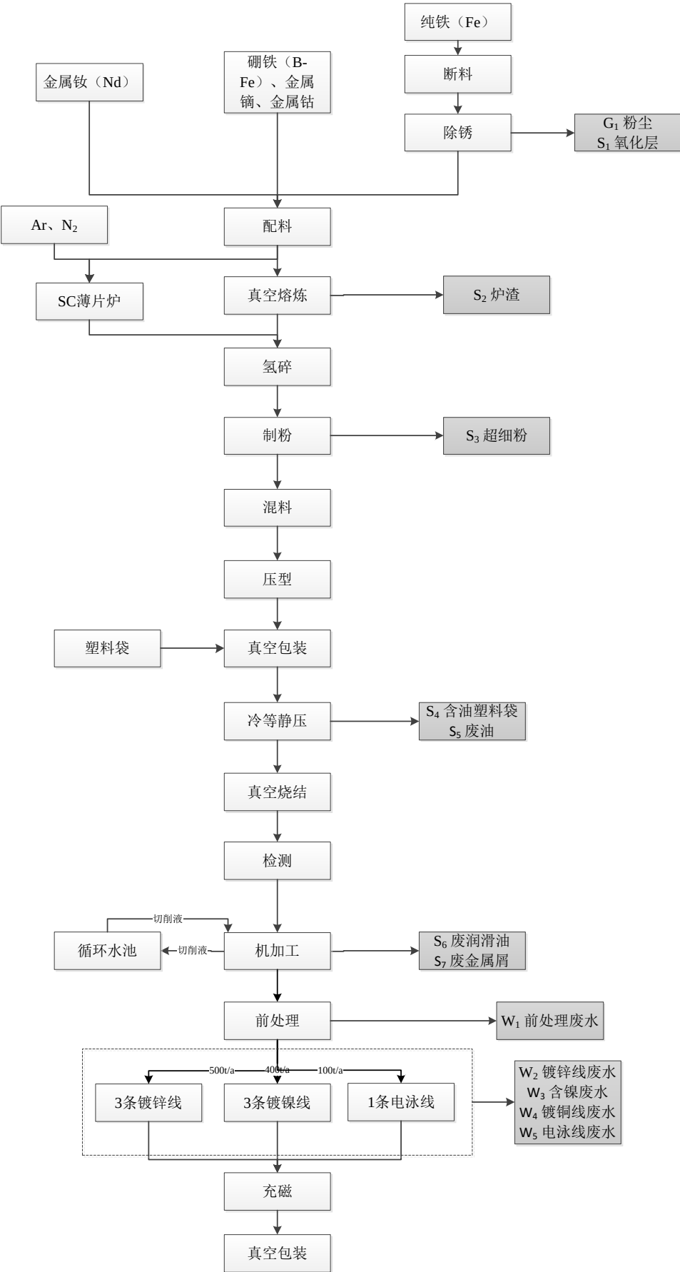
图 2-2 现有项目生产工艺流程及产污环节图
