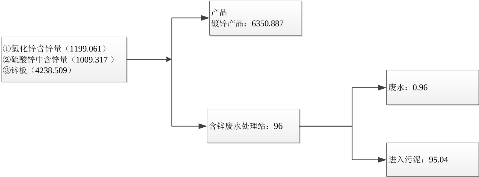
图 3-13 锌元素平衡图（单位：kg/a）
