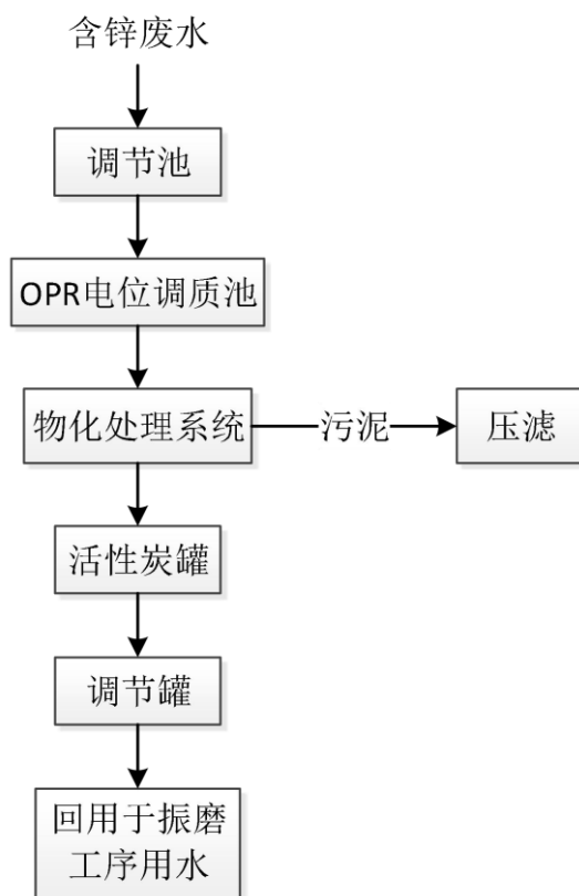
图 2-8 含锌废水处理工艺
