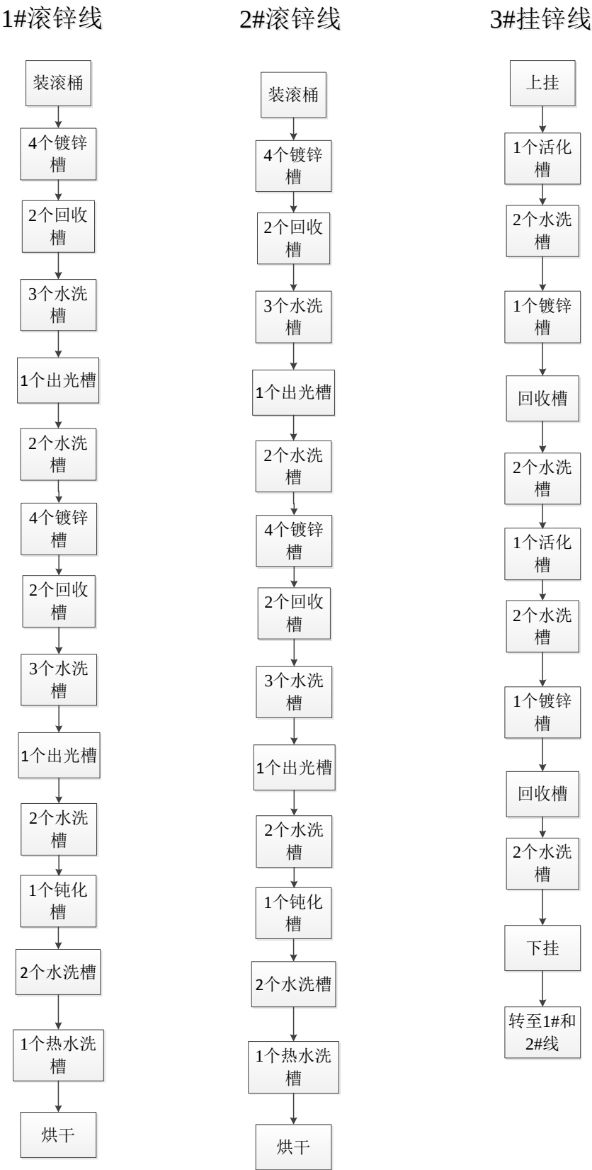
图 2-4 镀锌生产线生产工艺
