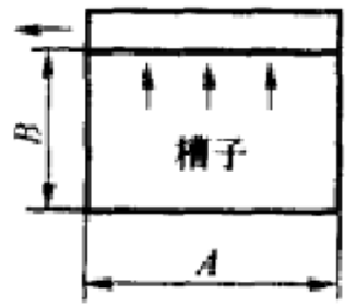
图 7-1 槽体单侧吸收罩布置示意图
