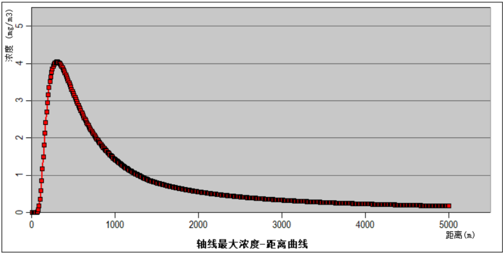
图 6-1 AFTOX 模型预测轴线/质心最大浓度-距离图
