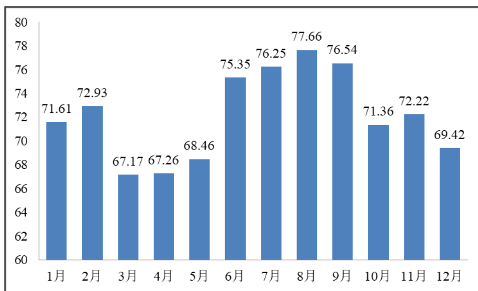
图 5-5 马鞍山累年月平均相对湿度（纵轴为百分比）
