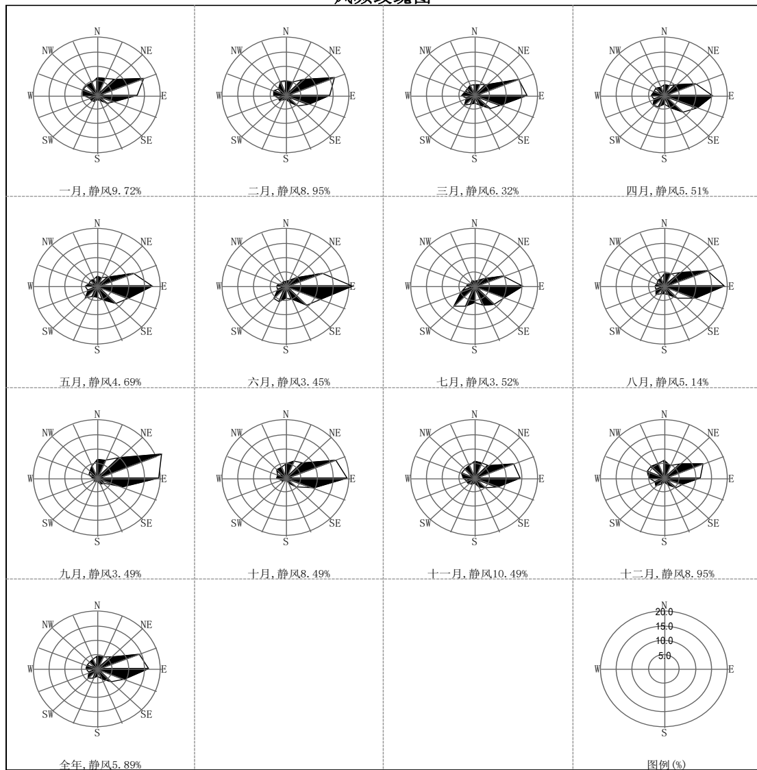
图 5-1 马鞍山月风向玫瑰图
