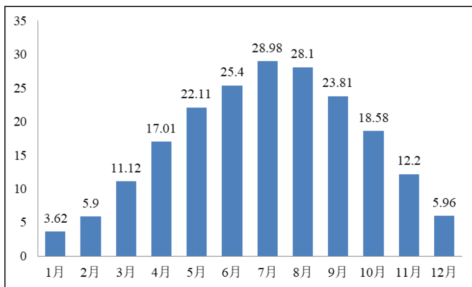
图 5-2 马鞍山累年月气温变化 (单位: °C)
