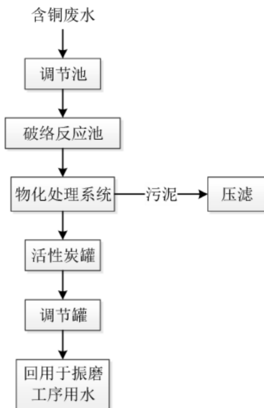
图 2-9 含铜废水处理工艺
